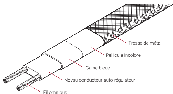
Composition du câble chauffant
