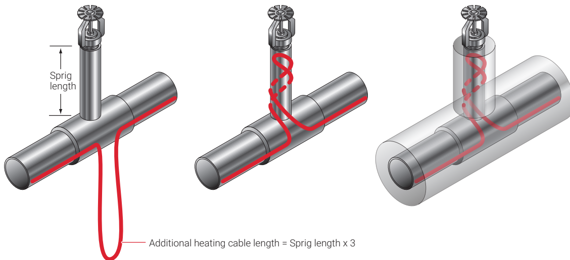
Fig. 14 XL-Trace Edge on sprinklers
