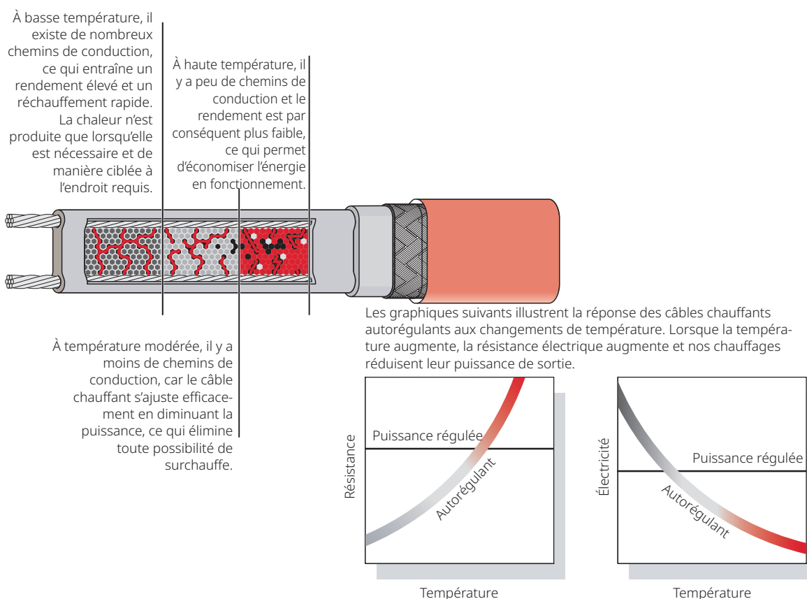
Fig. 2 Technologie du câble chauffant autorégulant
