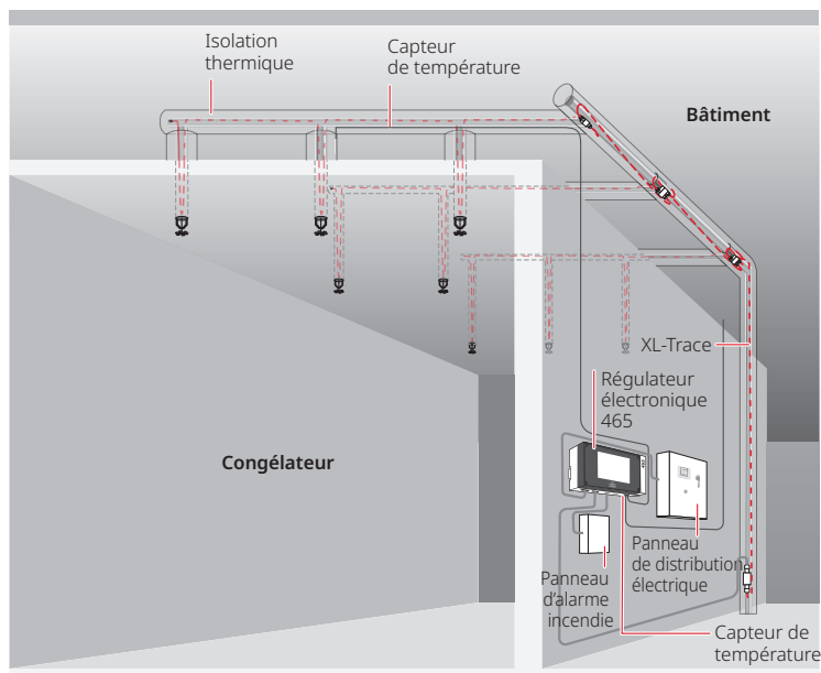
Fig. 8 Système d'extinction d'incendie caractéristique pour les applications dans des congélateurs
