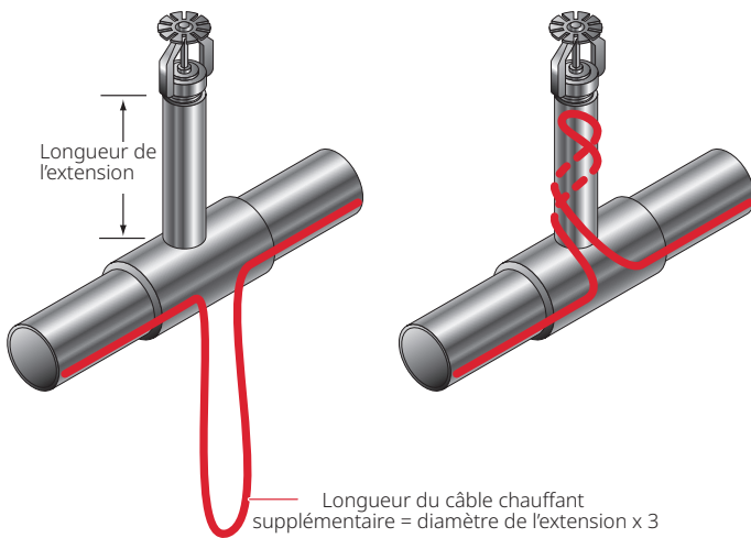
Fig. 14 Application XL-Trace pour les extincteurs automatiques
