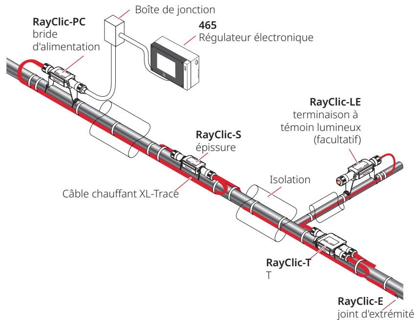
Fig. 4 Système caractéristique de canalisations en surface
