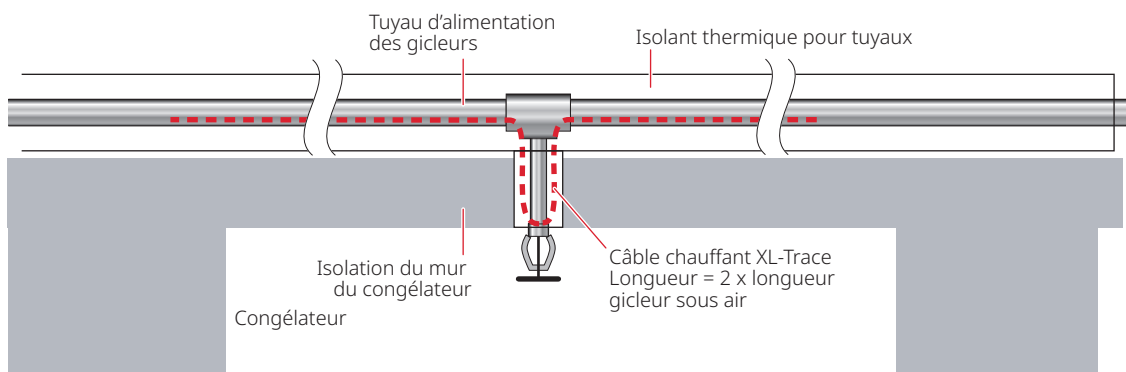
Fig. 15 XL-Trace sur les gicleurs avec extension orientés vers le bas
