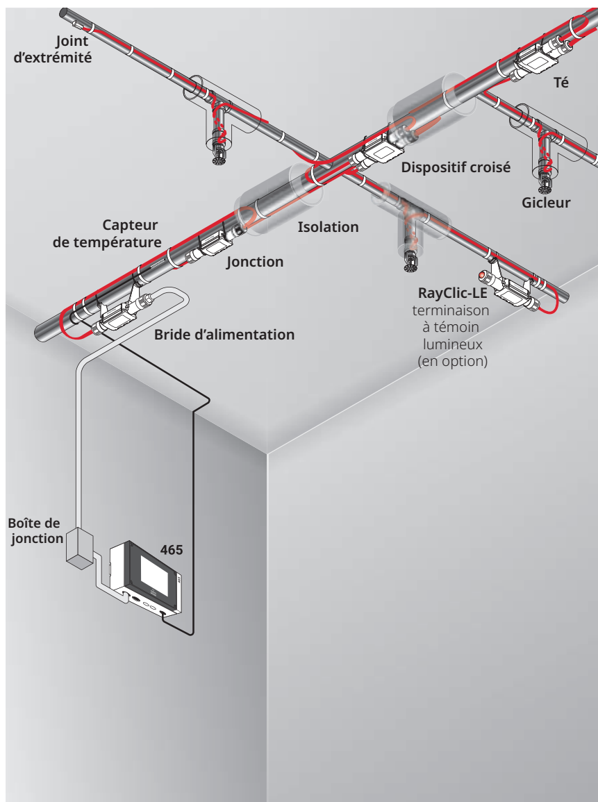
Fig. 12 Système de raccordement RayClic
