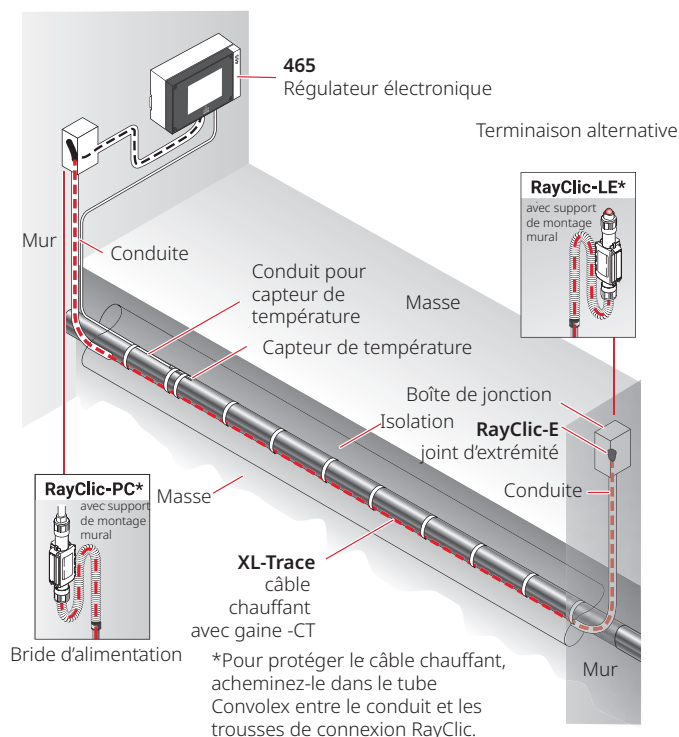
Fig. 13 Système caractéristique de canalisations enterrées
