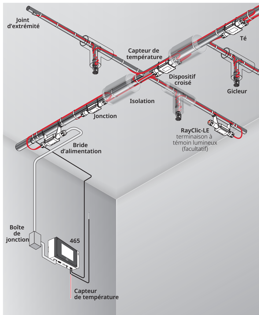
Fig. 7 Système d'extinction d'incendie caractéristique pour les embranchements munis d'extincteurs automatiques
