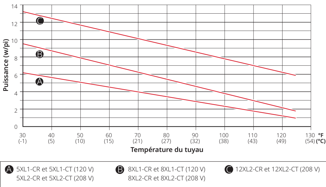
Fig. 11 Puissance de sortie du câble chauffant pour tuyau métallique
