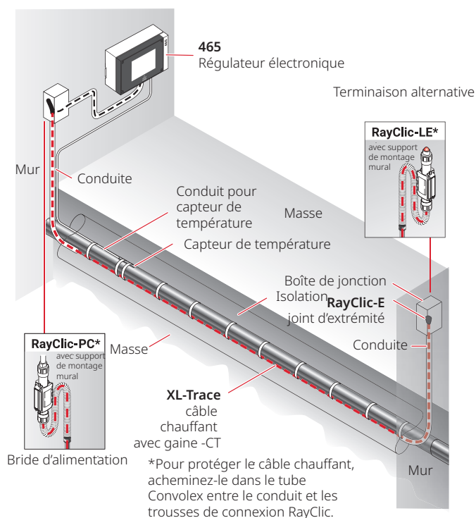
Fig. 5 Système caractéristique de tuyauterie enterrée
