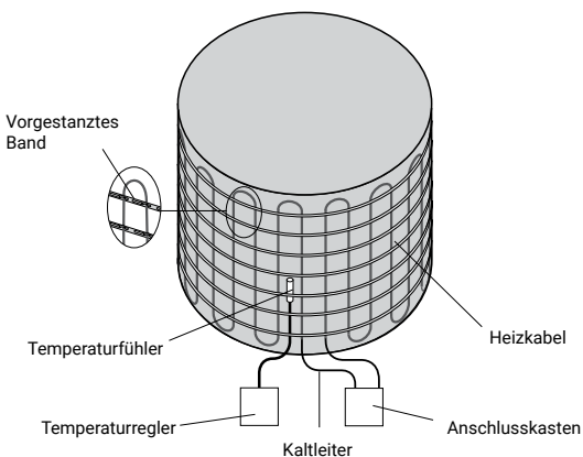
Abbildung 6: Befestigungselement: vorgestanztes Edelstahlband
