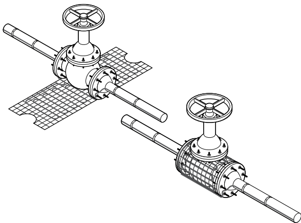
Abbildung 11-12: Heizkabel auf Metallgeflecht
