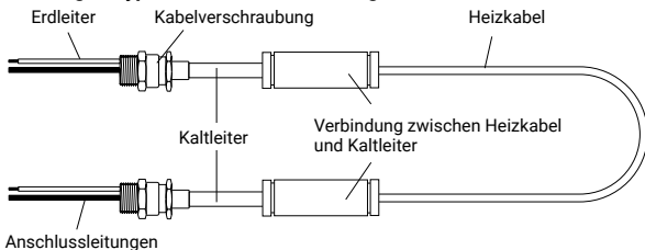
Abbildung 2: Typische Zusammenstellung der Heizelemente
