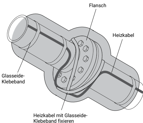
Abbildung 10: Typische Verlegung an Flanschen
