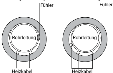
Abbildung 4: Kabelposition an Rohrleitung
