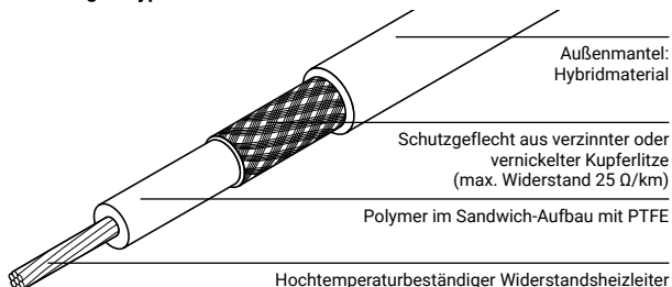
Abbildung 1: Typischer Kabelaufbau
