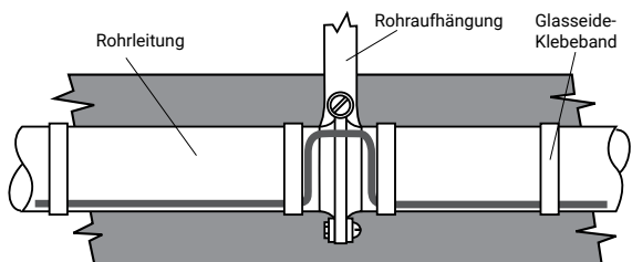
Abbildung 15: Heizkabelverlegung über Klemmen und Schellen
