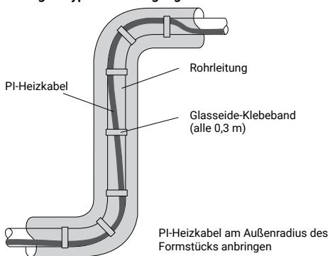
Abbildung 9: Typische Verlegung an Formstücken
