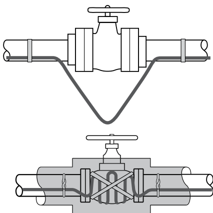
Abbildung 8: Typische Längenzugabe an Armaturen
