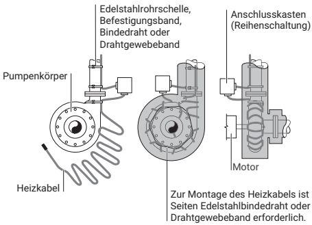
Abbildung 22: Pumpen
