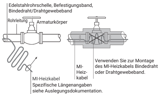
Abbildung 16b: Armaturen
