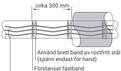
Figur 15: Fästa flera slag av kabel
