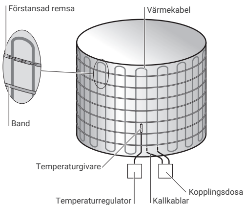
Figur 8: Fästordning: förstansat fästband
