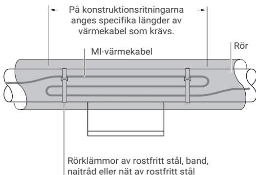
Figur 20: Stöd av typ rörsko och hylsa
