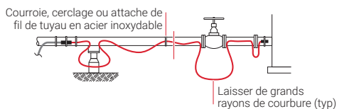
Figure 13 : Allocations pour vannes, brides, et supports de tuyau
