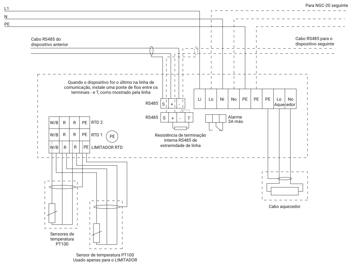
Figura 9: Diagrama de conexão elétrica NGC-20
