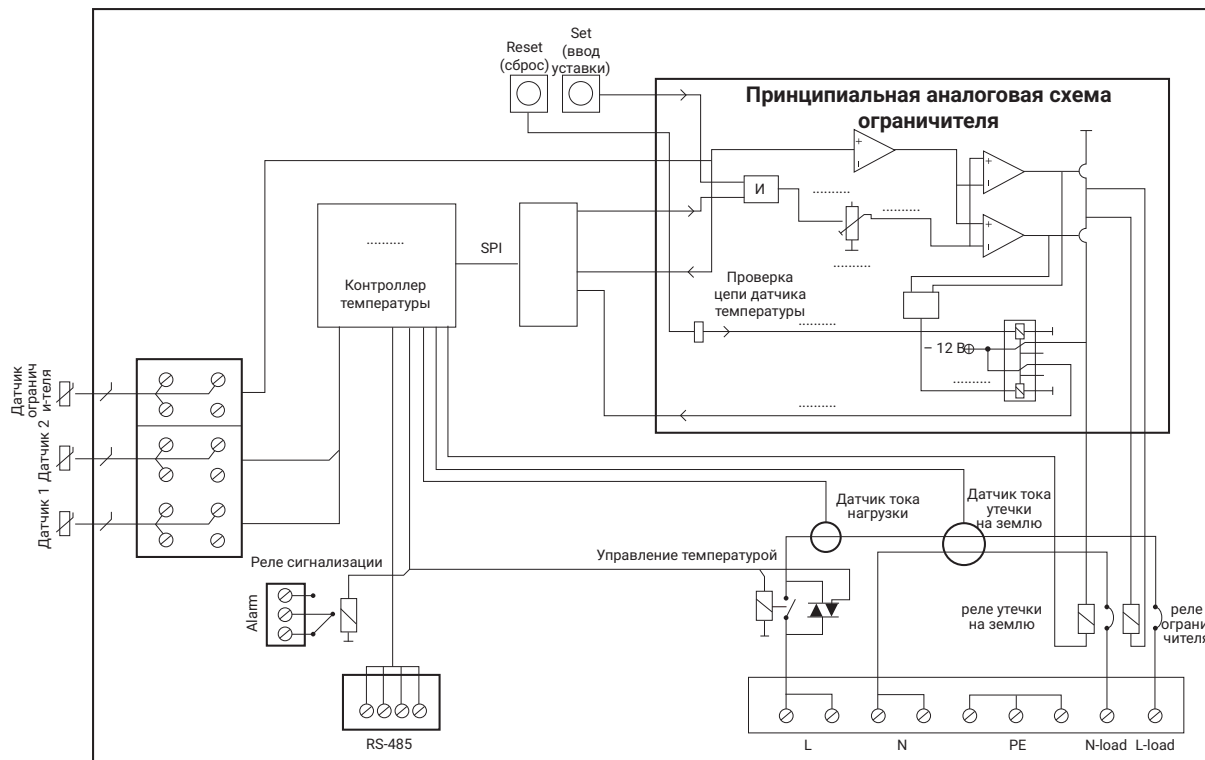
Рис. 10. Схема ограничителя температуры
