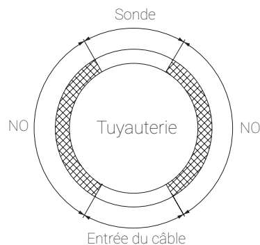
Figure 5: Montage d'une détection de température sur la tuyauterie
