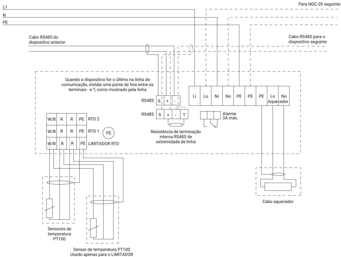
Figura 2: Diagrama de conexão NGC-20-C(L)-E
