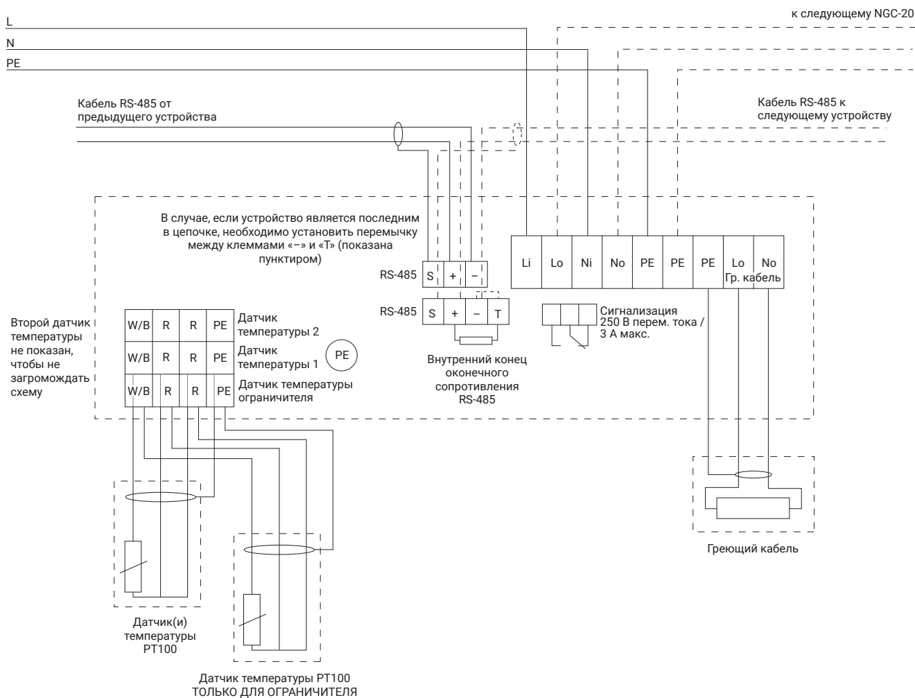
Рис. 2. Схема подключения NGC-20-C(L)-E
