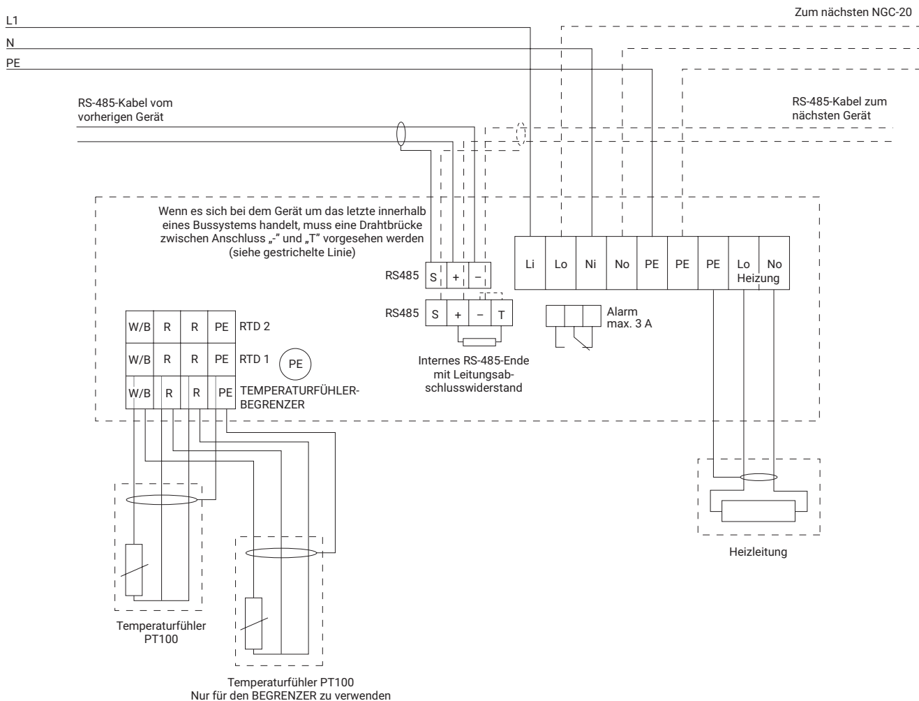
Abbildung 2: Anschlussdiagramm NGC-20-C(L)-E
