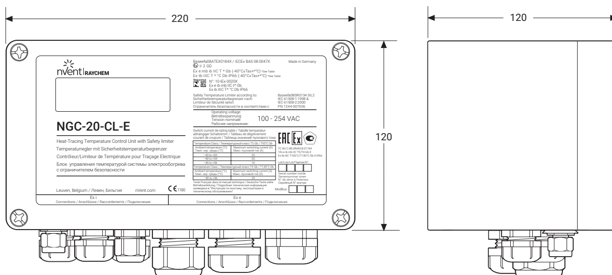
Рис. 1. Размеры NGC-20-C(L)-E
