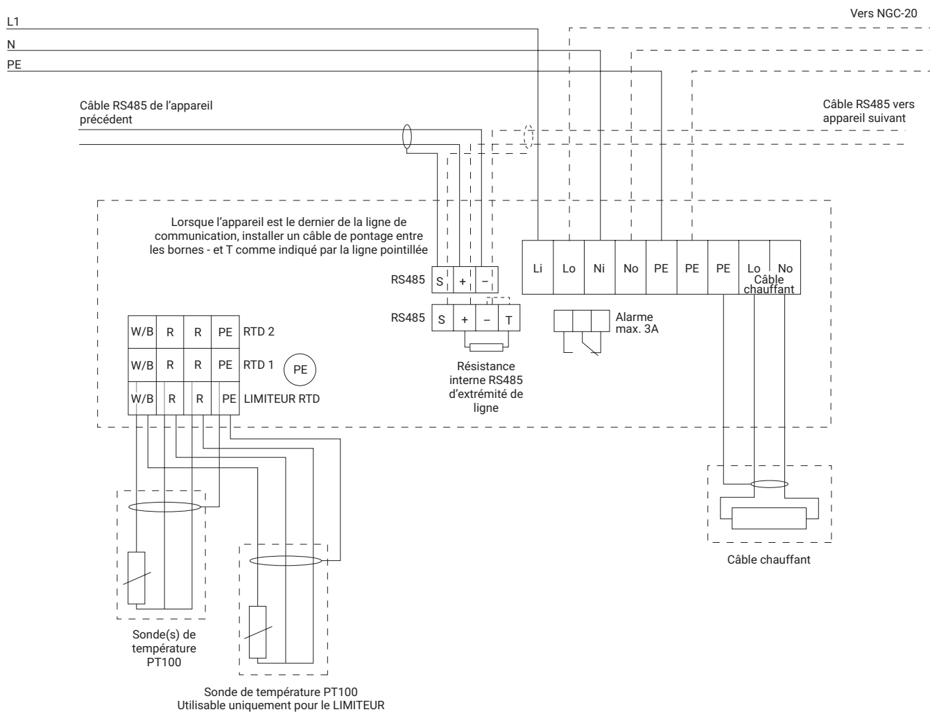
Figure 2: Schéma de câblage NGC-20-C(L)-E
