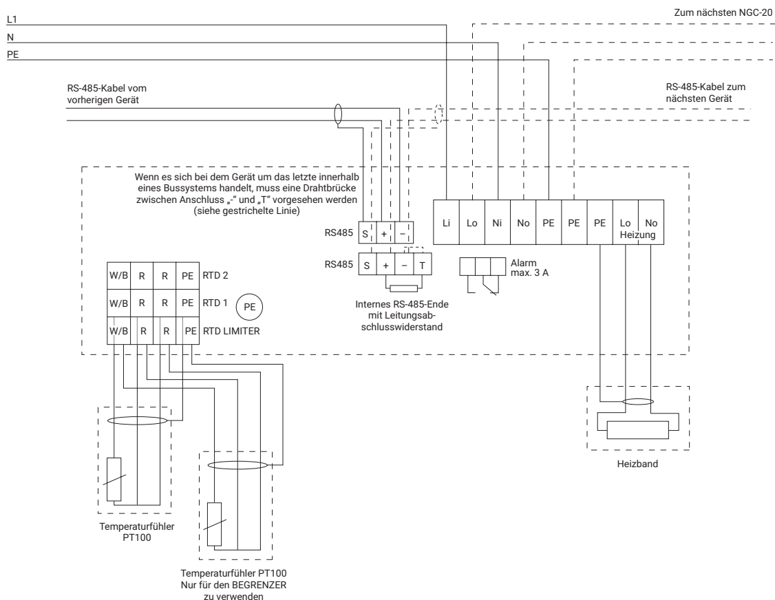
Abbildung 9: Elektrisches Anschlussdiagramm NGC-20
