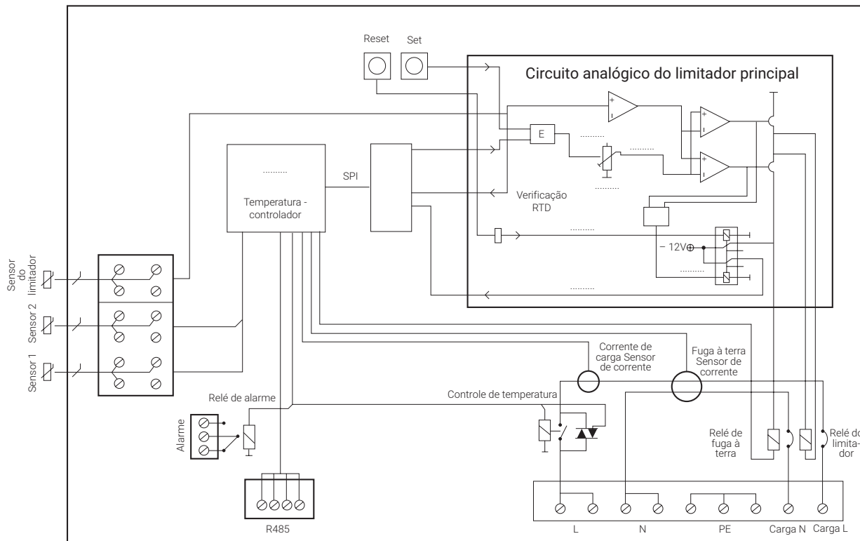
Figura 10: Diagrama de blocos do limitador
