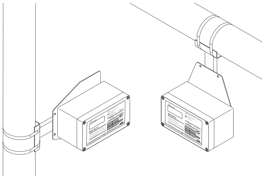
Рис. 4. Монтажные позиции для NGC-20
