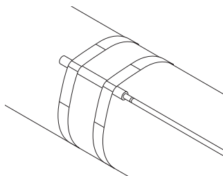
Montage de la sonde sur tuyau
