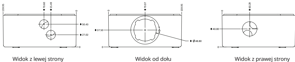
Rysunek 1: Miejsca wprowadzenia przewodów do obudowy Elexant 3500i
