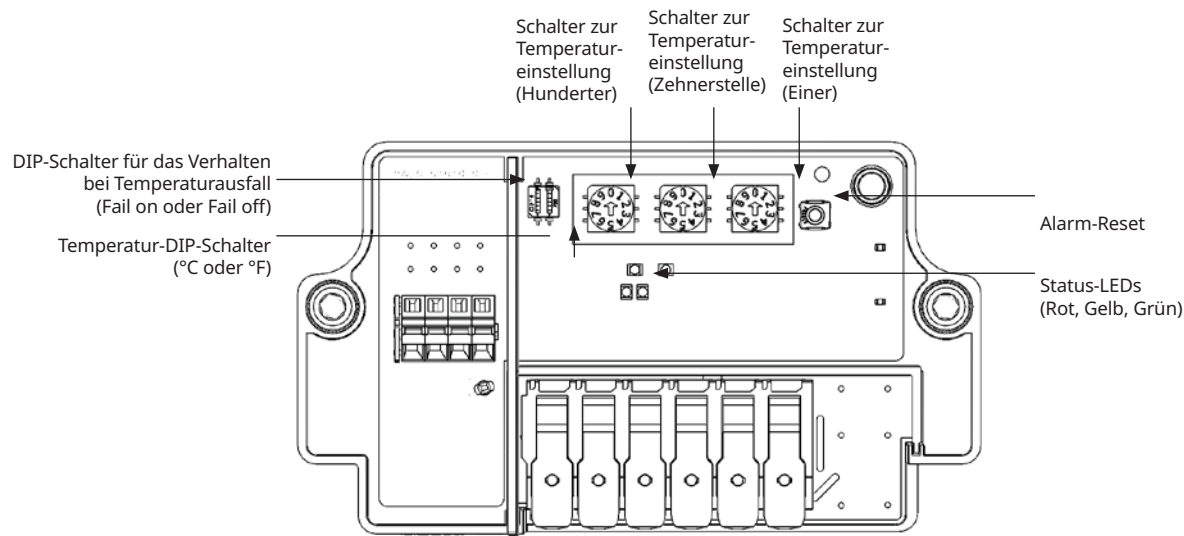
Abbildung 4: Digitale Schalter und Drehregler der Elexant 3500i bei Standard- und Alarmausführung
