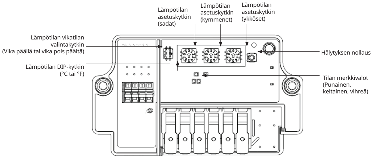
Kuva 4: Elexant 3500i -mallin vakioversion ja hälytysversion digitaaliset kytkimet ja kiertokytkimet
