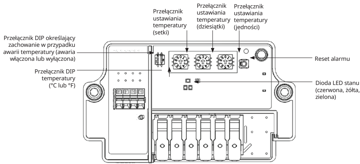
Rysunek 4: Przełączniki cyfrowe i pokręteła wariantu standardowego i alarmowego Elexant 3500i
