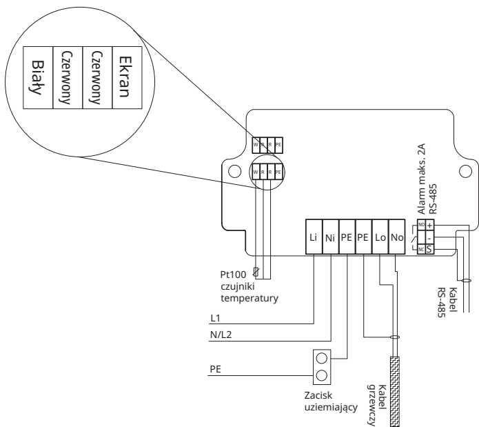
Rysunek 2: Schemat połączeń
