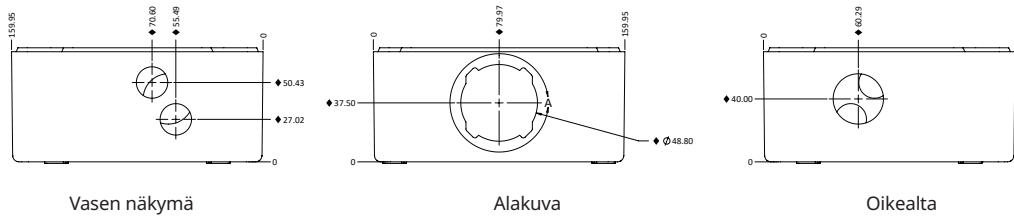
Kuva 1: Elexant 3500i -keskittimen liitännäpaikat
