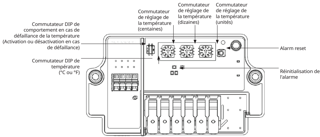
Figure 4 : Commutateurs numériques et boutons rotatifs de l'Elexant 3500i en version standard et avec alarme
