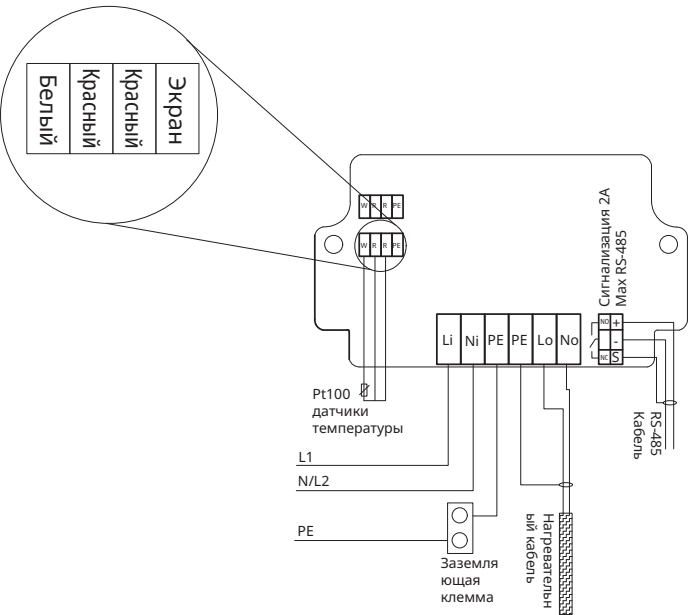
Рисунок 2: Схема подключения
