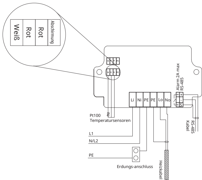
Abbildung 2: Schaltplan
