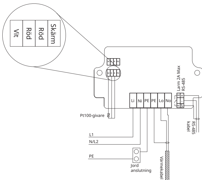
Figur 2: Kopplingsschema
