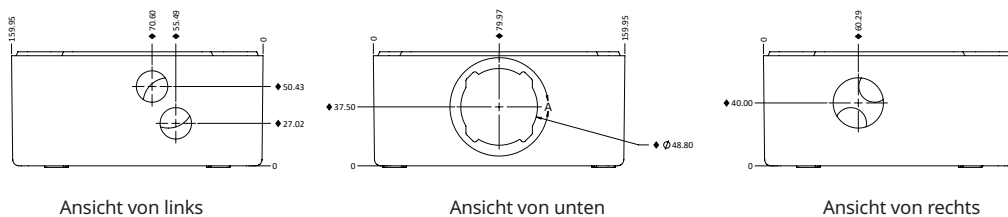
Abbildung 1: Einführungsstellen für den Elexant 3500i-Hub
