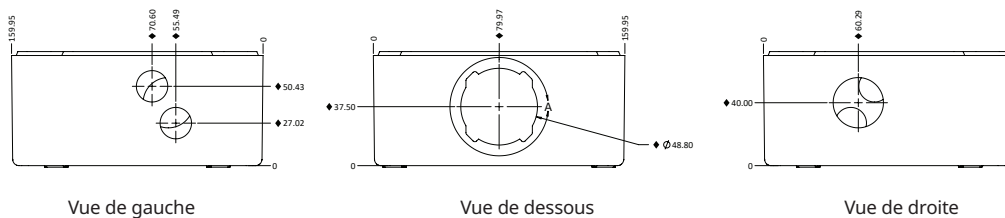
Figure 1 : Emplacements d'entrée du concentrateur Elexant 3500i
