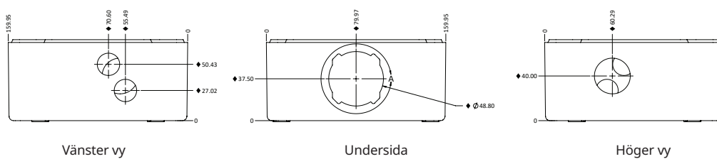
Figur 1: Placering av genomföringar för Elexant 3500i
