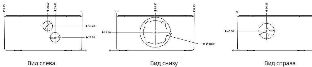
Рисунок 1: Расположение точек ввода кабеля Elexant 3500i
