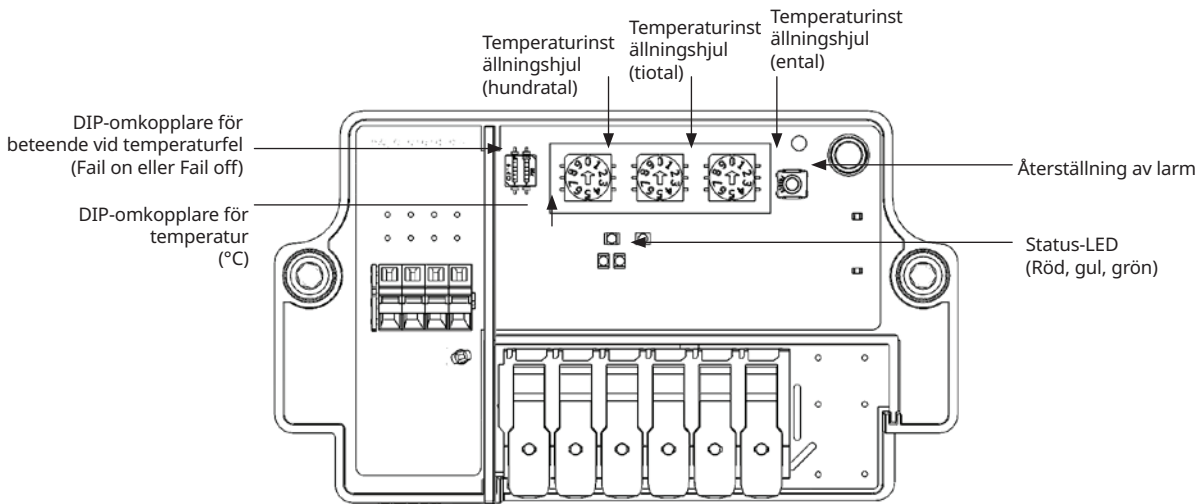
Figur 4: Elexant 3500i standard- och larmvariantens digitala omkopplare och vridreglage
