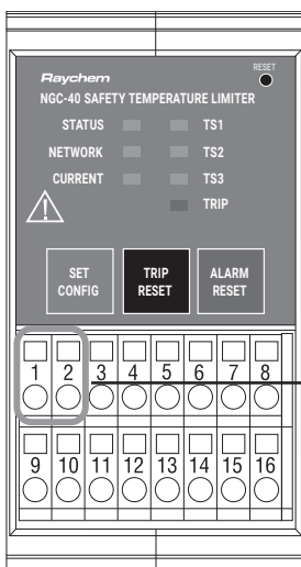
Abbildung 5: Schütz-Anschlussklemmen
