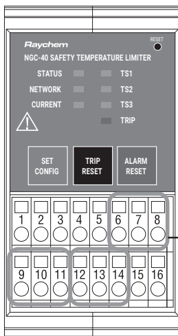
Abbildung 4: Anschluss der Temperaturfühler
