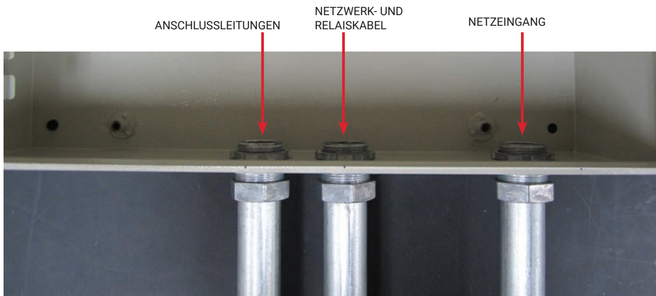
Abbildung 3: Beispiel für fertige Durchführungen
