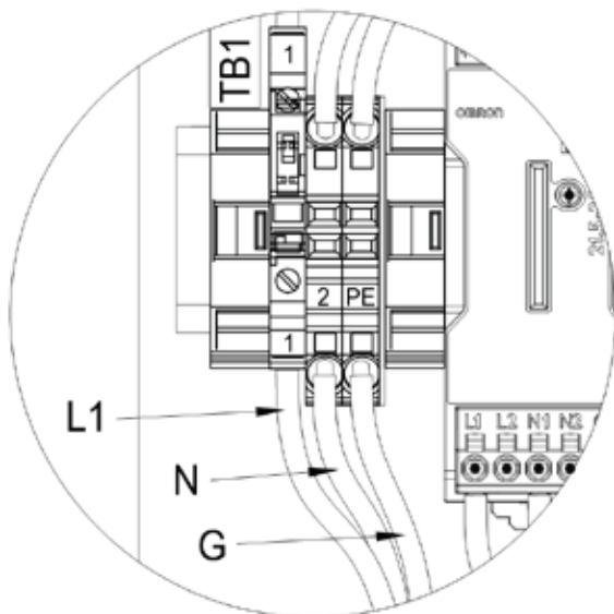
Abbildung 2 - Spannungsversorgung
